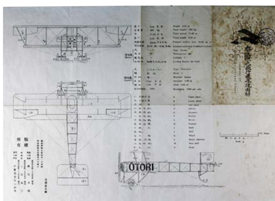
⑤ 453 奈良原式飛行機鳳凰号図解 55×39cm 明治45 一〇、〇〇〇円(税込一一、〇〇〇円)
